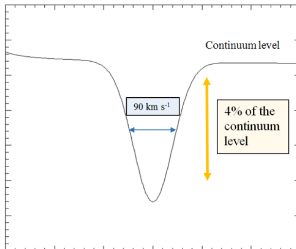
Fig. 1. Линия поглощения HI 21 см по отношению к излучению радиогалактики в континууме
