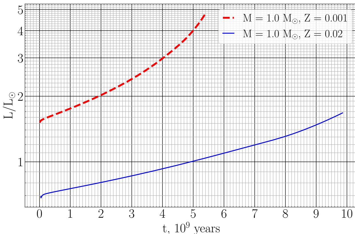
Рис. 1: Светимость звезд с массой 1 M_{\odot} на стадии главной последовательности, Z – металличность звезды
